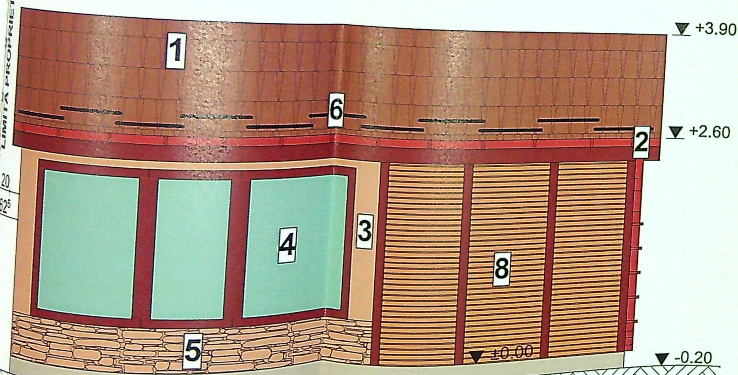
FATADA NORD-EST
