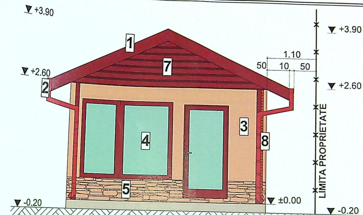
FATADA NORD-VEST
